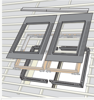
Kettős összeépítés EKY segédszarufával BDX –K– 2011E
