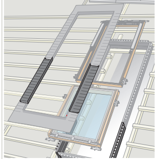
Beépítés kiegészítő elemmel GIL/GIU BDX WK34 2011
