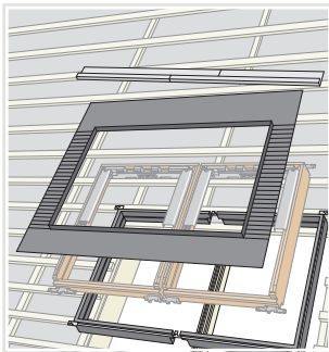
Kettős összeépítés EBY segédszarufával BDX –K– 2011
