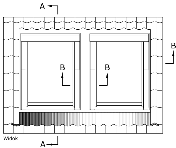
Przekrój A-A 1:5
