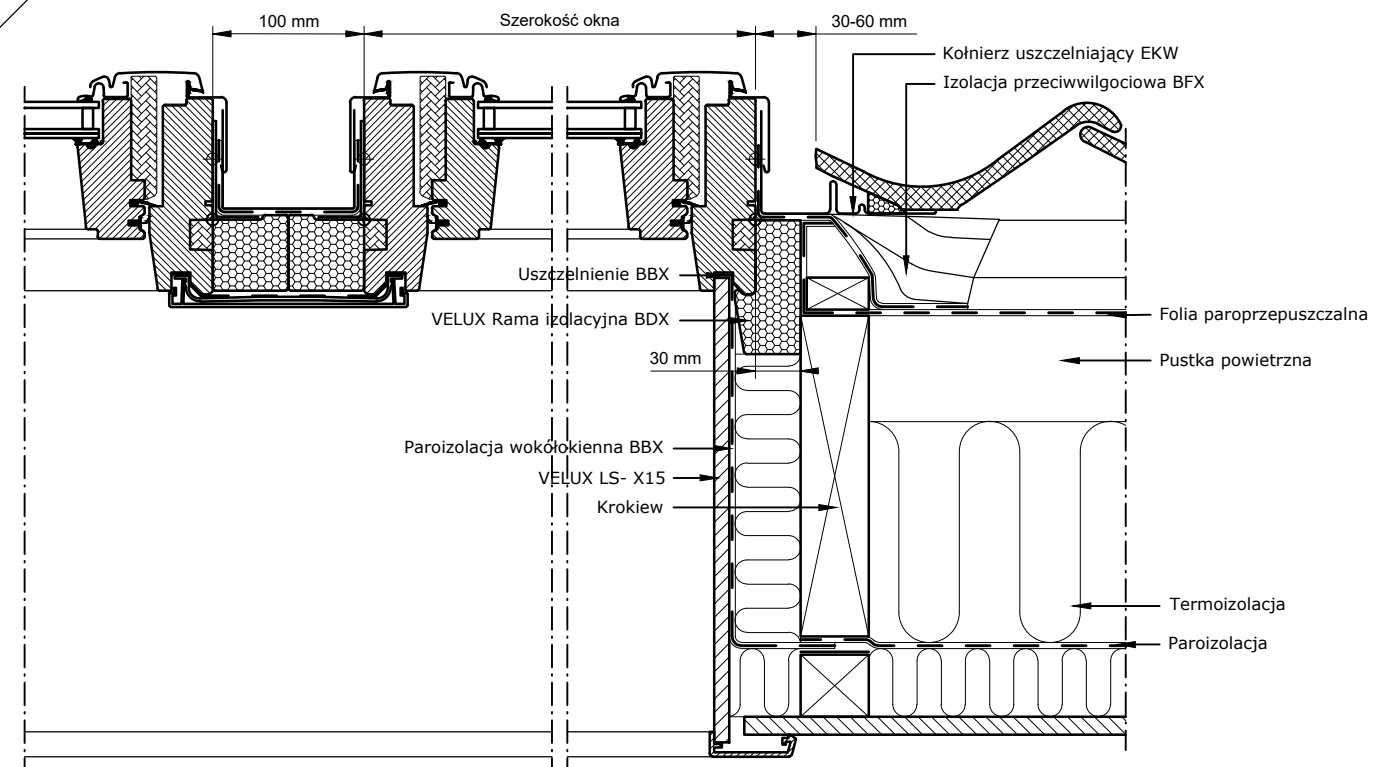
Przekrój B-B 1:5
