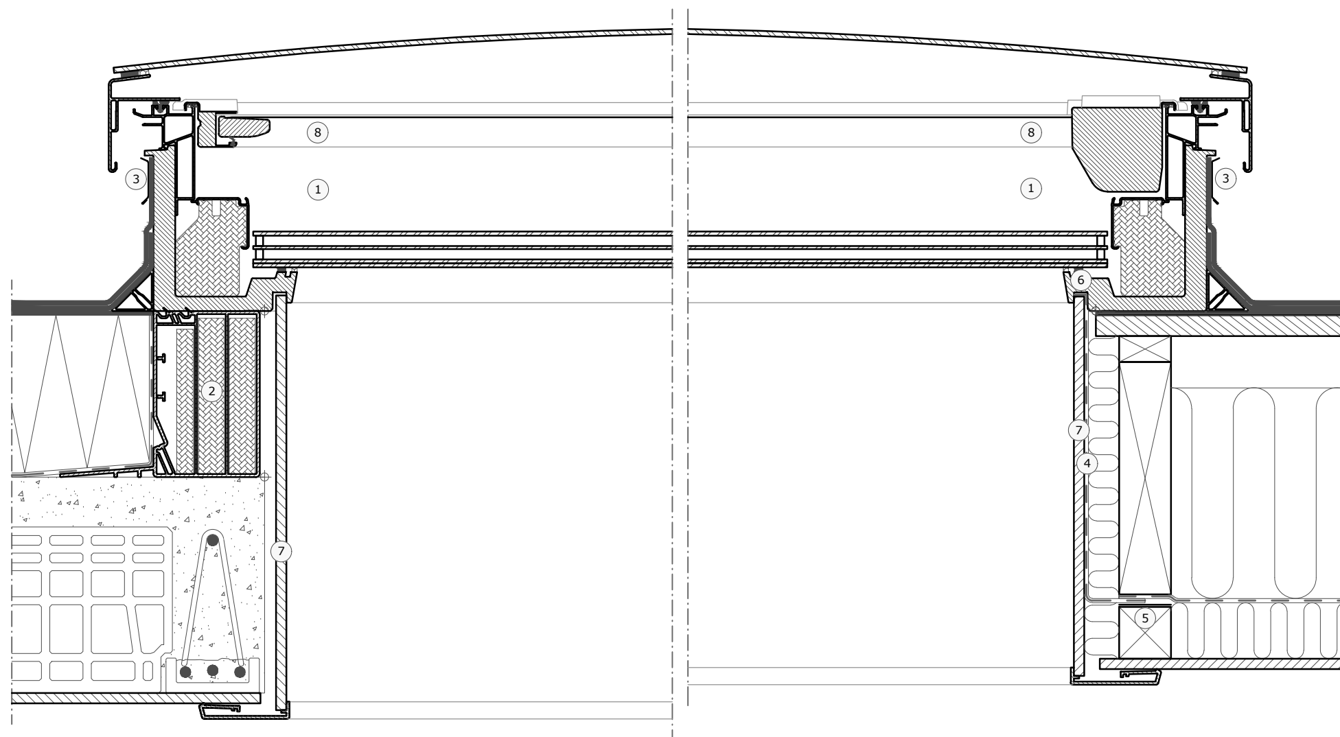
Presek A-A 1:5
