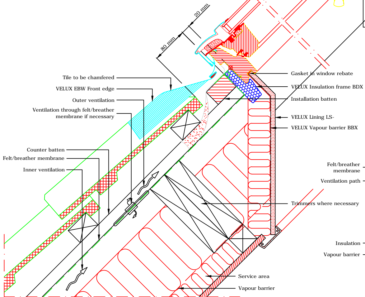
Section A-A 1:5
